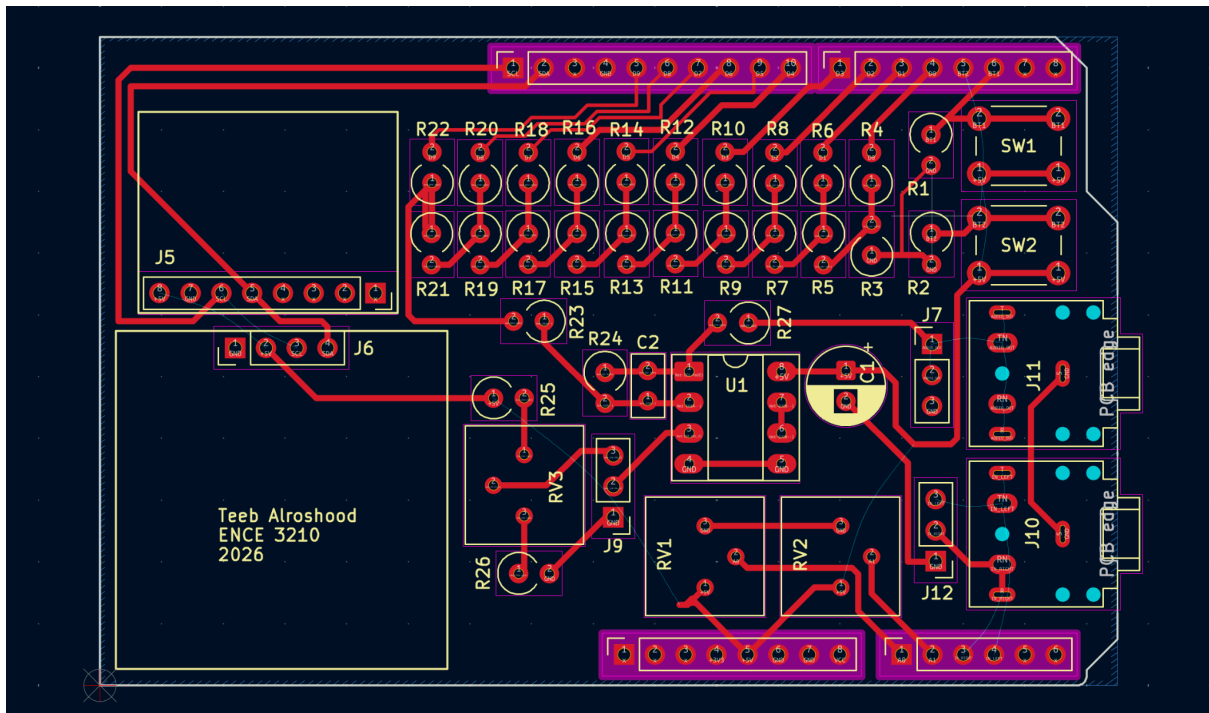
PCB front:
